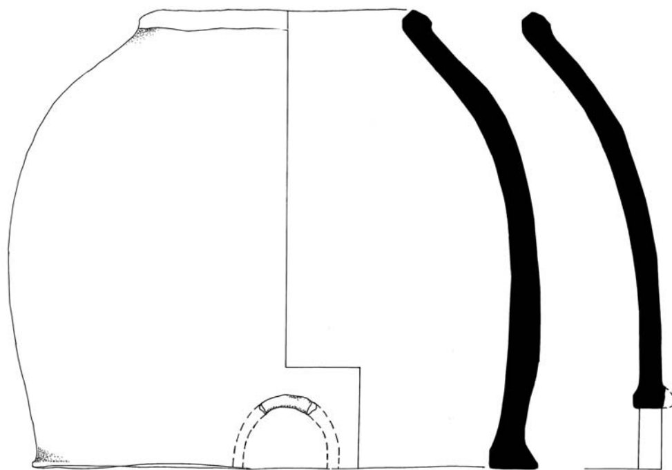
איור 2 (למעלה): התנור מתל רחוב לאחר שחזורו במכון לארכאולוגיה באוניברסיטה העברית בירושלים איור 3 (למטה): התנור מתל רחוב, שרטוט חתך
